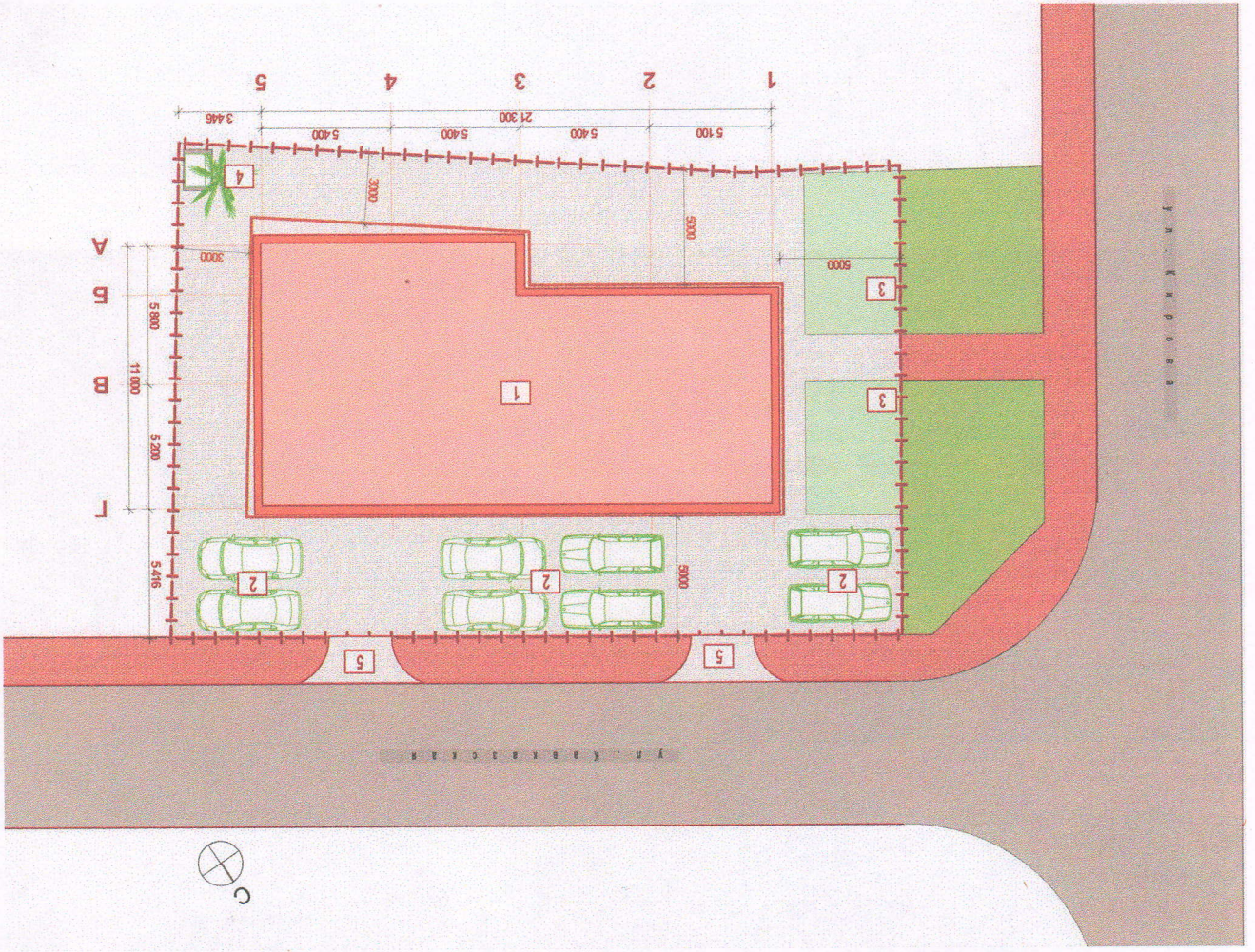
Технико-эксплуатационная организационная схема земельного участка
